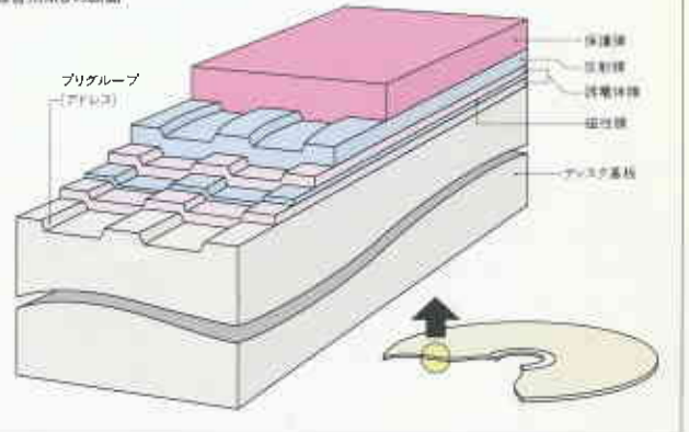
録音用MDの断面
