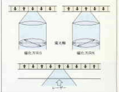
録音用MDの再生原理
