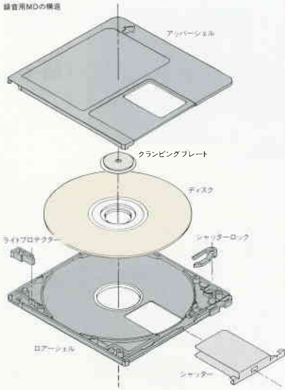
録音用MDの構造
